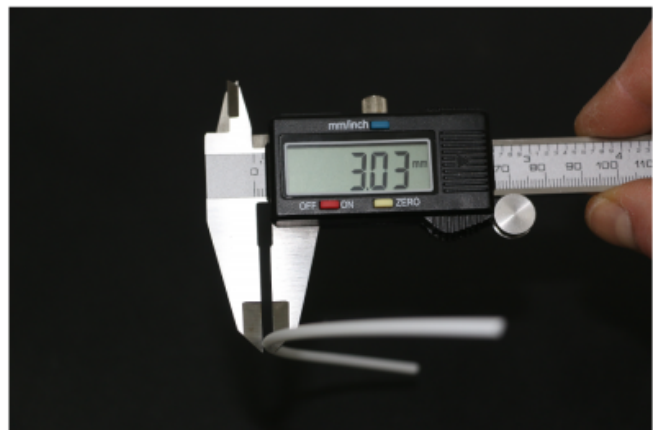
☐ Dieselbe Stelle, um 90° versetzt gemessen. Der Durchmesser überschreitet die zulässige Toleranz – das Filament ist unrund und muss ersetzt werden.
