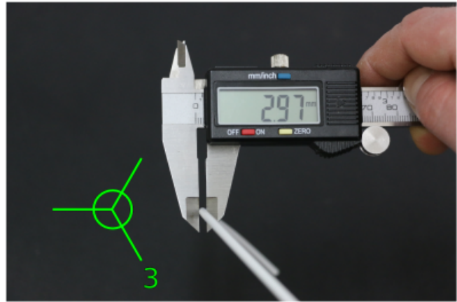
☐ Dritter zu messender Durchmesser – das dargestellte Filament überschreitet die Toleranzen und muss ersetzt werden.
