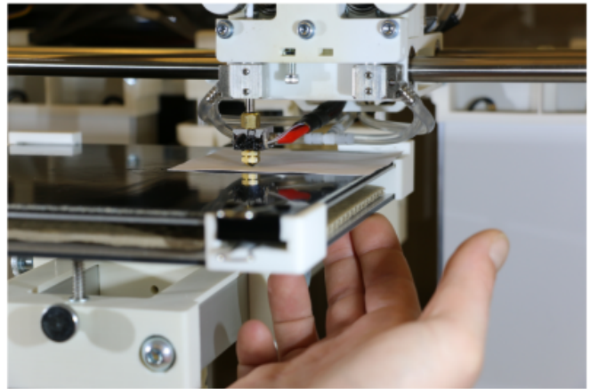
Manuelles Leveln mit Papier als Distanzhalter – vorderer und hinterer rechter Leveling-Punkt.
