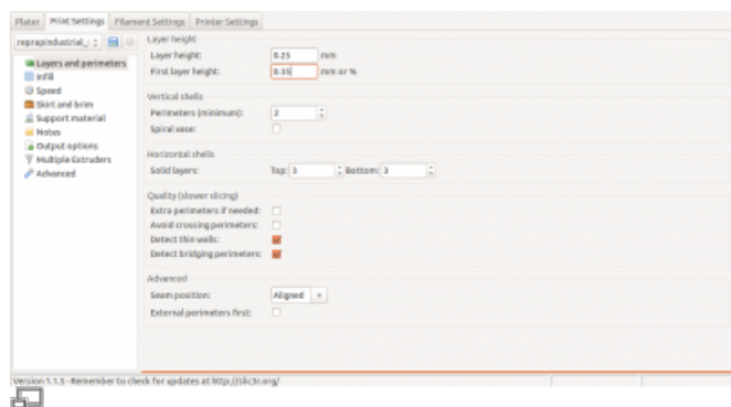
Slic3r Print Settings – Dicke der ersten Schicht einstellen.
