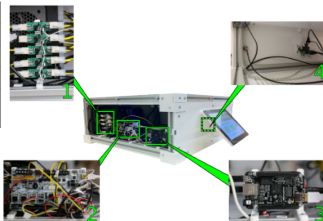
Linke Innenansicht der Elektronikkammer.
