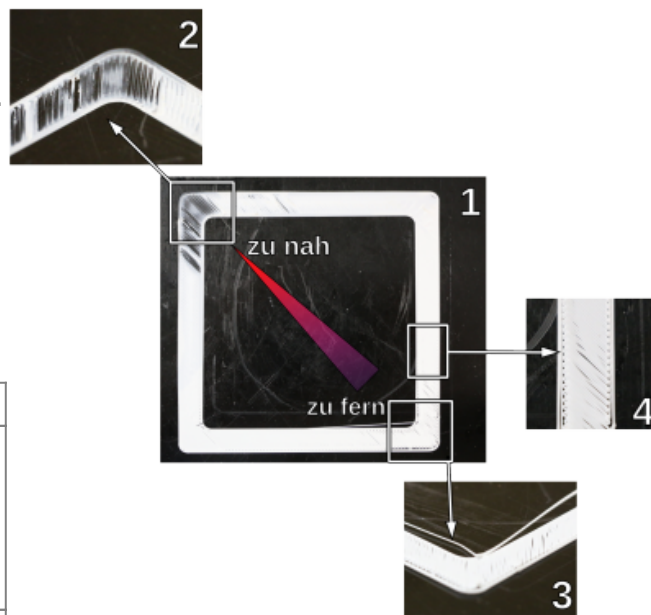
Levelingfehler: Beispiele für charakteristische Erscheinungsbilder der ersten Schicht.
